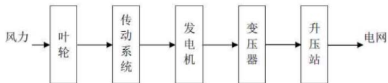
图 4-4 营运期工艺流程及产污环节图
